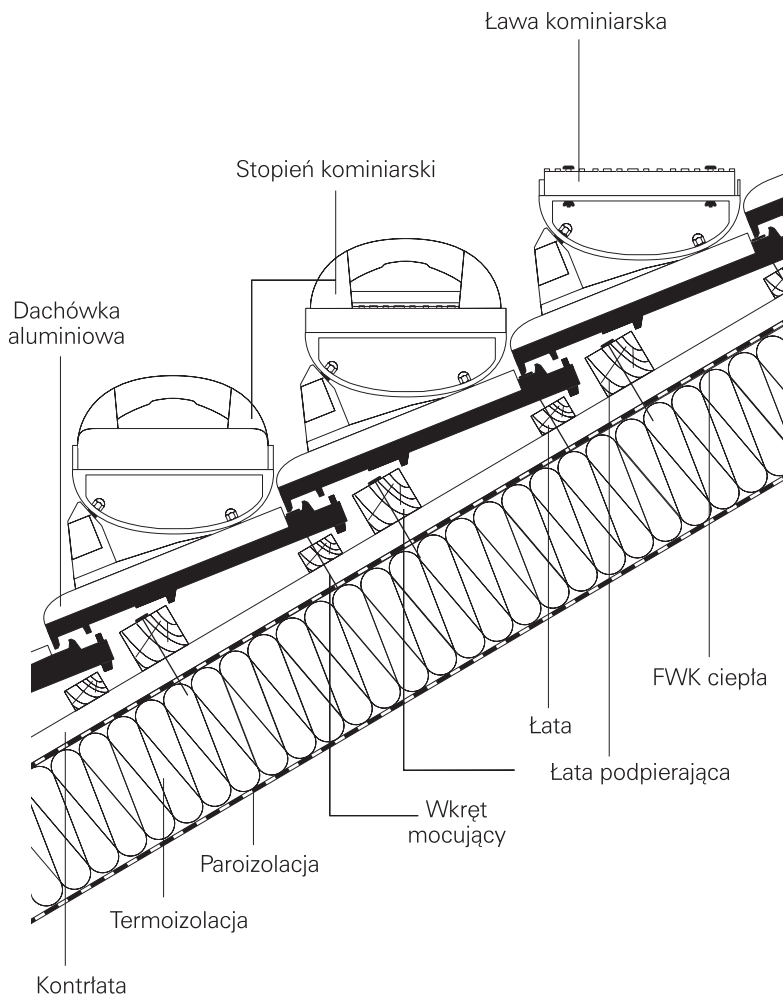
Rysunki detali – Komunikacja na dachu
