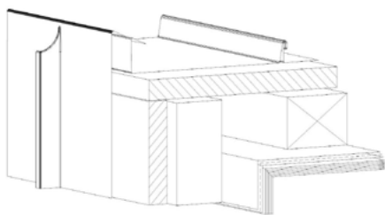
Detal: połączenie elewacji na rąbek z dachem
