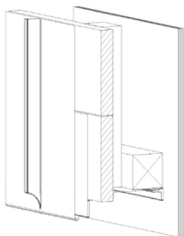
Detal: zakończenie elewacji na rąbek
