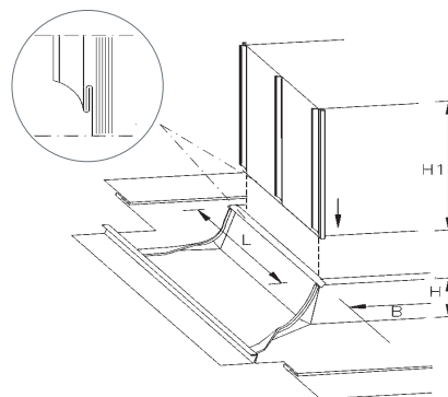
Detal: przykładowa obróbka komina
