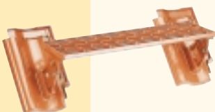
Alu-Standrost komplett mit 2 Grundpfannen
